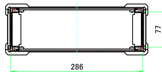
A-A (1:5)
