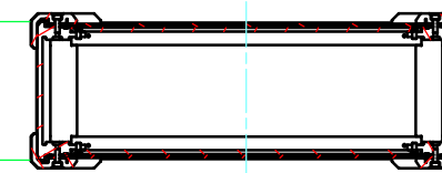
D-D (1:6)
