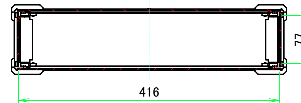
A-A (1:6)
