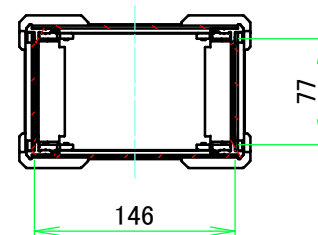
A-A ( 1 : 5.5 )
