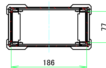
A-A ( 1 : 5.5 )
