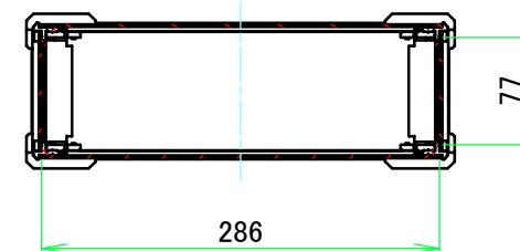
A-A (1:6)
