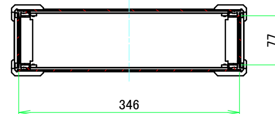
A-A (1:6)
