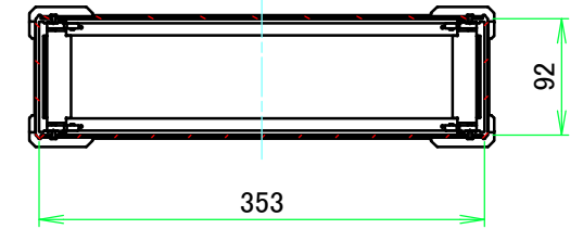
C-C ( 1 : 6.5 )
