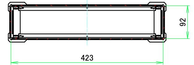
C-C ( 1 : 6.5 )
