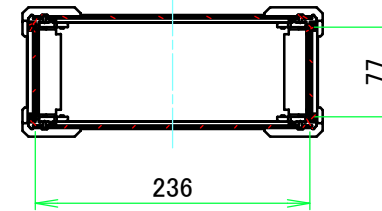
A-A ( 1 : 6.5 )
