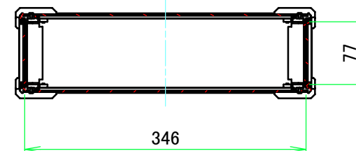
A-A (1:6.5)
