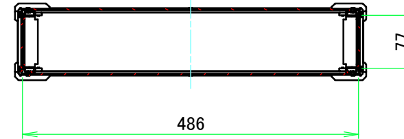
A-A ( 1 : 7.5 )
