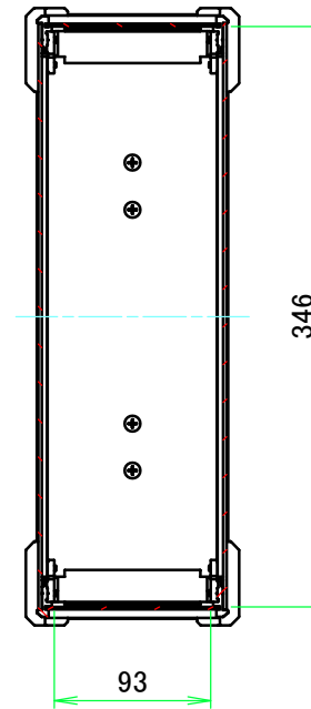
A-A (1:5)
