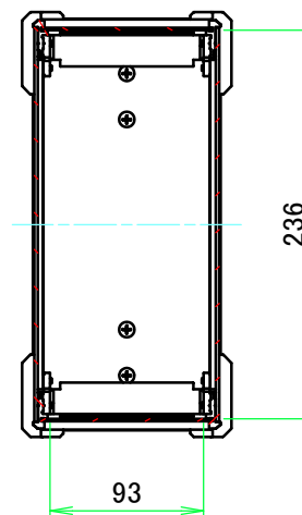
A-A (1:5)
