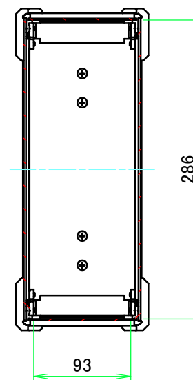
A-A (1:5)
