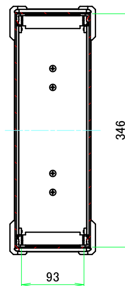
A-A ( 1 : 5.5 )
