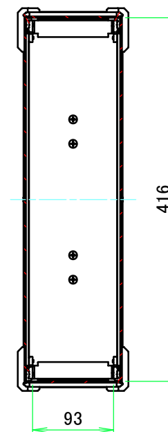
A-A (1:6)
