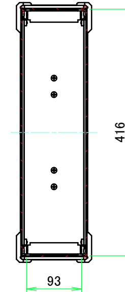
A-A ( 1 : 6.5 )
