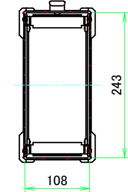
C-C ( 1 : 6.5 )
