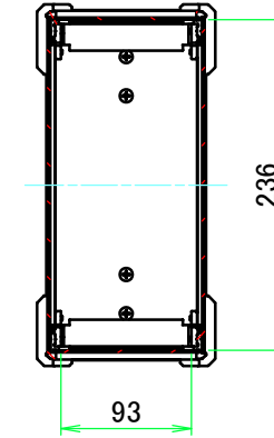
A-A (1:6)
