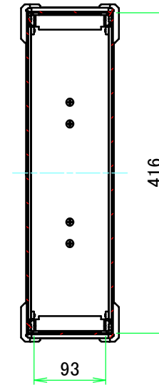
A-A (1:7)
