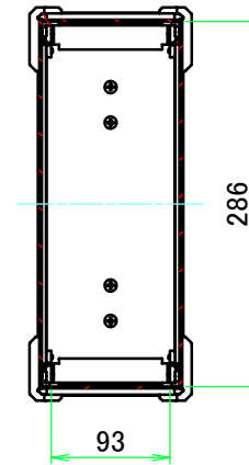
A-A (1:6.5)
