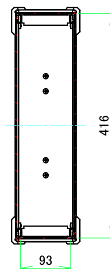
A-A (1:7)
