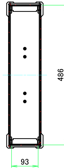
A-A (1:8)
