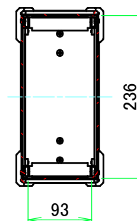
A-A ( 1 : 7.5 )
