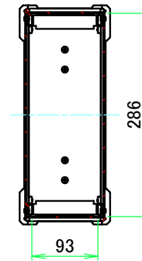
A-A (1:7.5)
