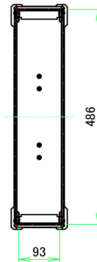
A-A (1:8.5)
