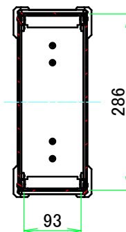
A-A ( 1 : 8.5 )
