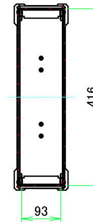
A-A (1:9)
