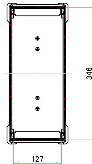
A-A (1:6)
