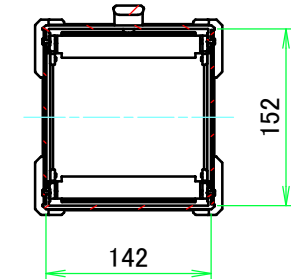
C-C ( 1 : 6.5 )
