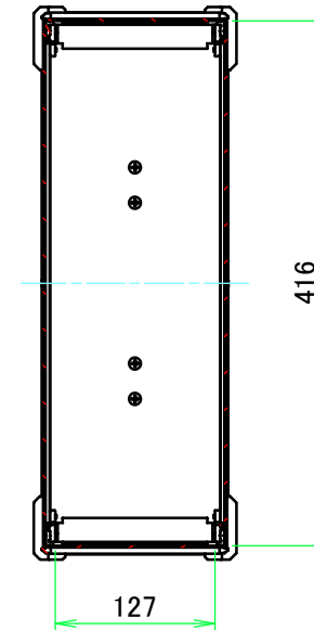
A-A ( 1 : 6.5 )
