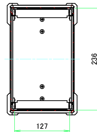
A-A (1:5)
