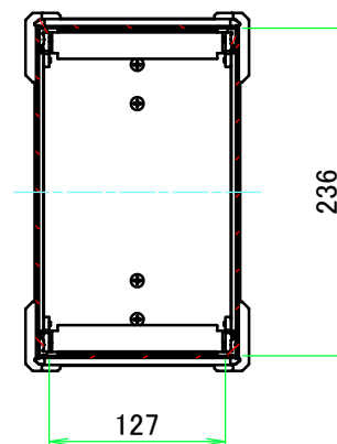
A-A (1:6)
