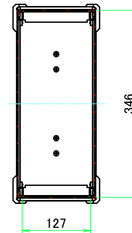
A-A (1:7)
