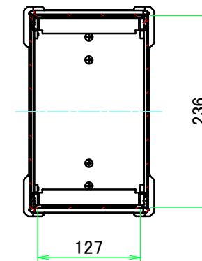
A-A ( 1 : 6.5 )
