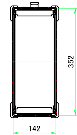
C-C ( 1 : 7.5 )
