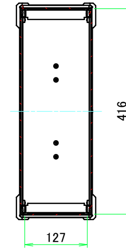
A-A ( 1 : 7.5 )
