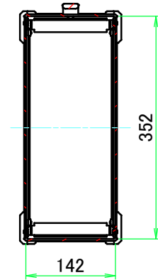
C-C ( 1 : 8.5 )
