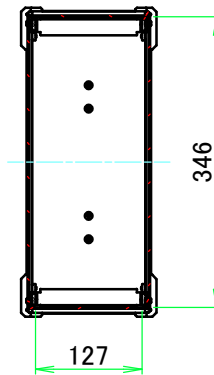
A-A (1:9)
