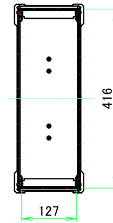
A-A (1:9)
