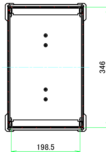
A-A ( 1 : 6.5 )
