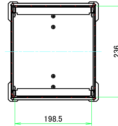
A-A (1:6)
