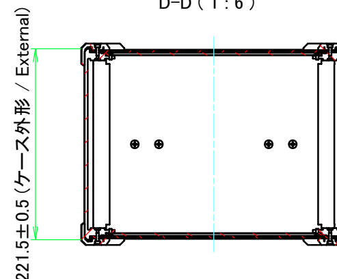
D-D (1:6)
