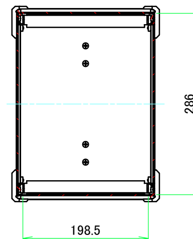
A-A (1:6)
