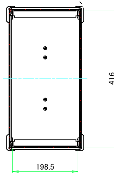
A-A (1:7)
