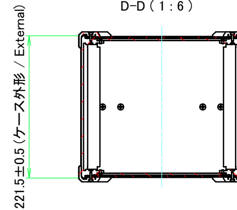
D-D (1:6)
