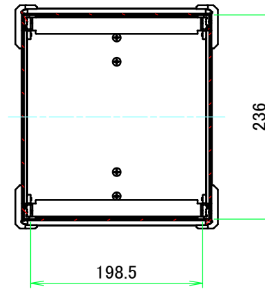
A-A (1:6)
