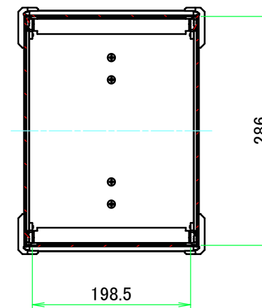
A-A (1:6.5)
