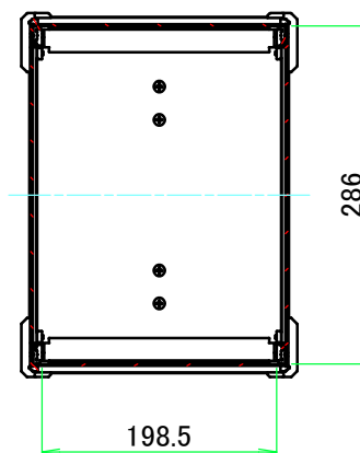
A-A (1:7)
