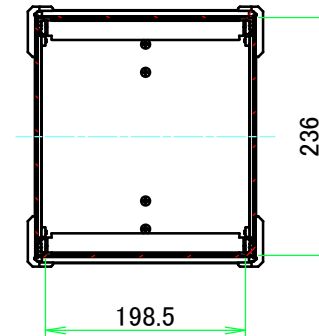
A-A (1:7.5)
