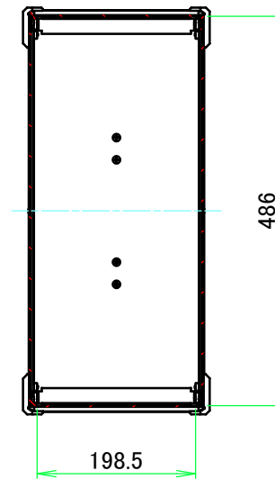
A-A (1:8.5)
