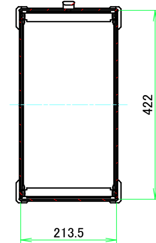
C-C ( 1 : 8.5 )
