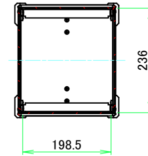
A-A ( 1 : 8.5 )
