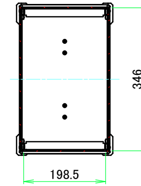
A-A (1:9)
