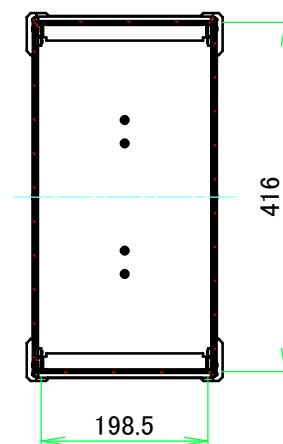
A-A (1:9)
