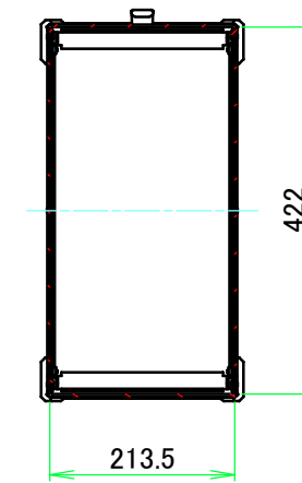
C-C ( 1 : 9.5 )
