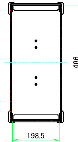
A-A ( 1 : 9.5 )
