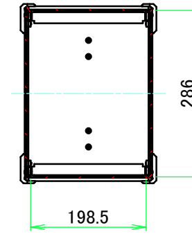
A-A (1:9)
